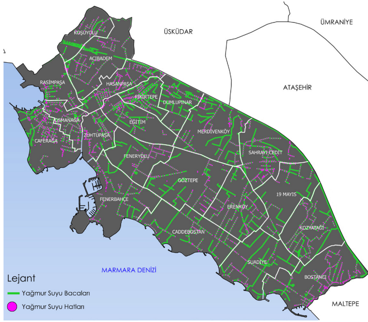
Harita 84: Kadıköy İlçesi'nde Yer Alan Mevcut Yağmur Suyu Altyapısı
