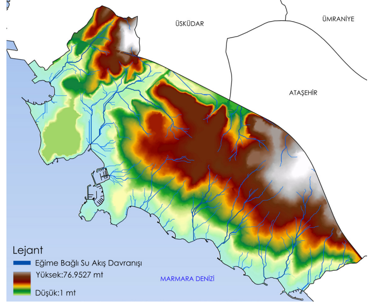
Harita 19: Eğime Bağlı Su Akış Davranışı
