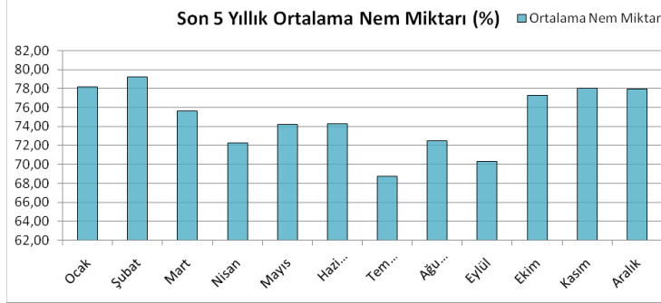
Grafik 6: Kadıköy İlçesi'nin Son 5 Yıllık Ortalama Nem Miktarının Aylara Göre Dağılımı
