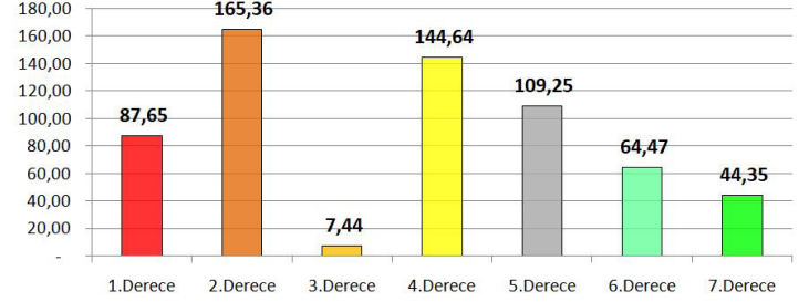
Grafik 7: Doğal Afet Riski Altındaki Alanların Dağılımı
